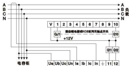
JKW6接线图
